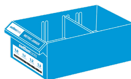
Dimensions of Drawer: 70mm (H) x 90mm (W) x 218mm (D)
